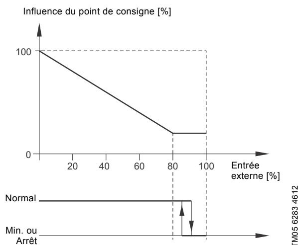
Fig. 74 "Inverse avec Arrêt" et "Inverse avec Min."
