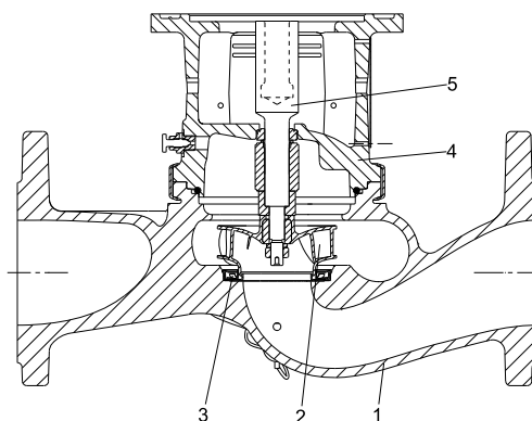
Fig. 28 Schéma en coupe d'une pompe TPE2
