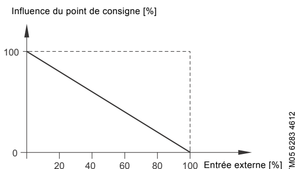
Fig. 73 Fonction inverse
