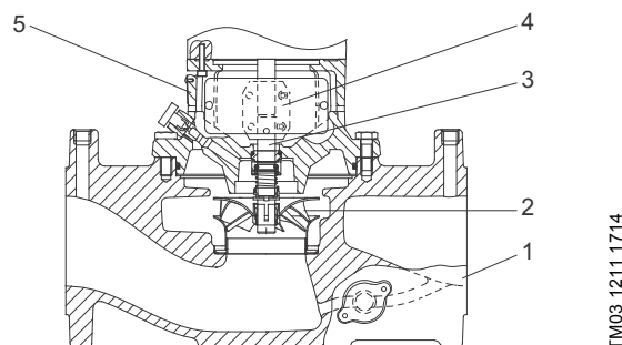
Fig. 11 Schéma en coupe des pompes TP Série 200 (avec bride)
