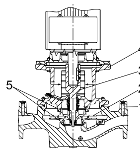
Fig. 13 Schéma en coupe des pompes TP Série 300
