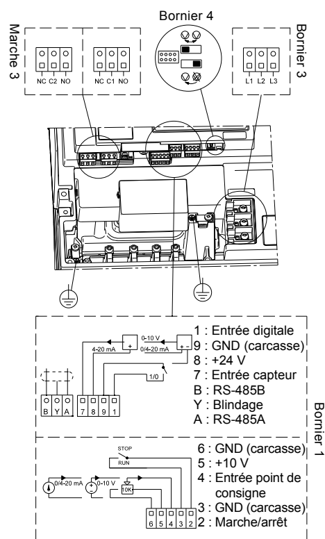
Fig. 110 Bornes, TPED Série 2000
