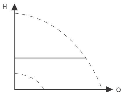
Fig. 54 Pression constante
