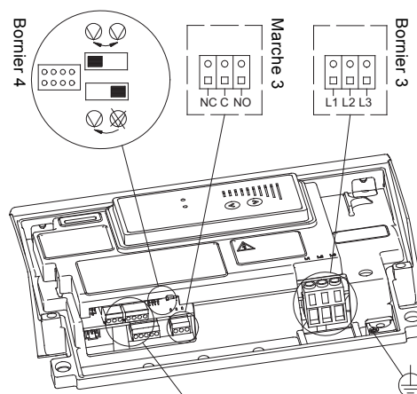
Fig. 106 Bornes de connexion
