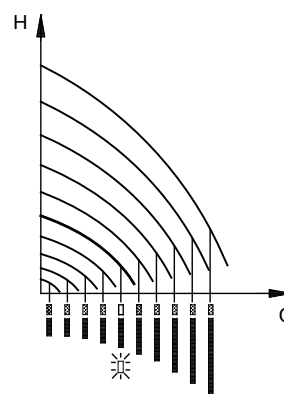
Fig. 37 Réglage du rendement de la pompe, mode de régulation "Courbe constante"
