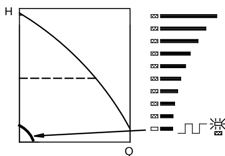
Fig. 39 Courbe mini
