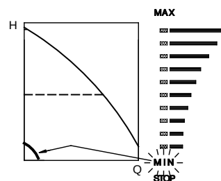
Fig. 45 Courbe mini
