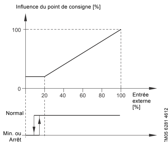
Fig. 72 "Linéaire avec Arrêt" et "Linéaire avec Min."
