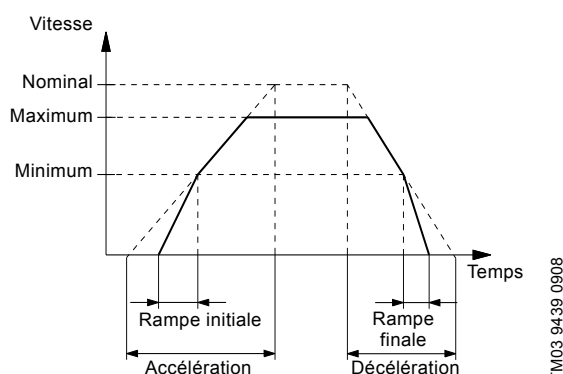
Fig. 79 Accélération et décélération
