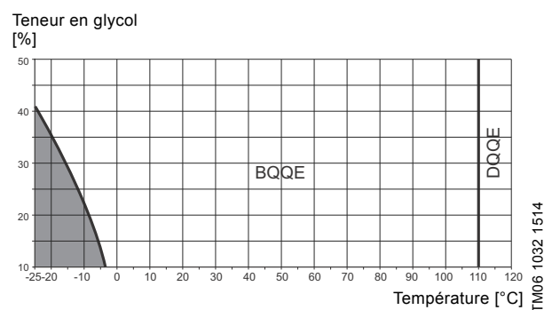
Fig. 7 Plage de service des garnitures mécaniques EPDM
