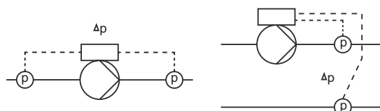
Fig. 59 Pression différentielle constante
