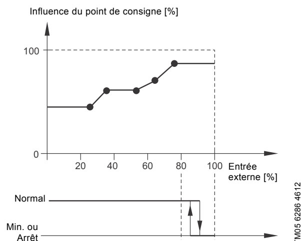
Fig. 77 Tableau d'influence avec Arrêt au Max.
