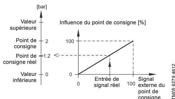
Fig. 70 Exemple de l'influence du point de consigne
