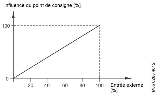
Fig. 71 Fonction linéaire
