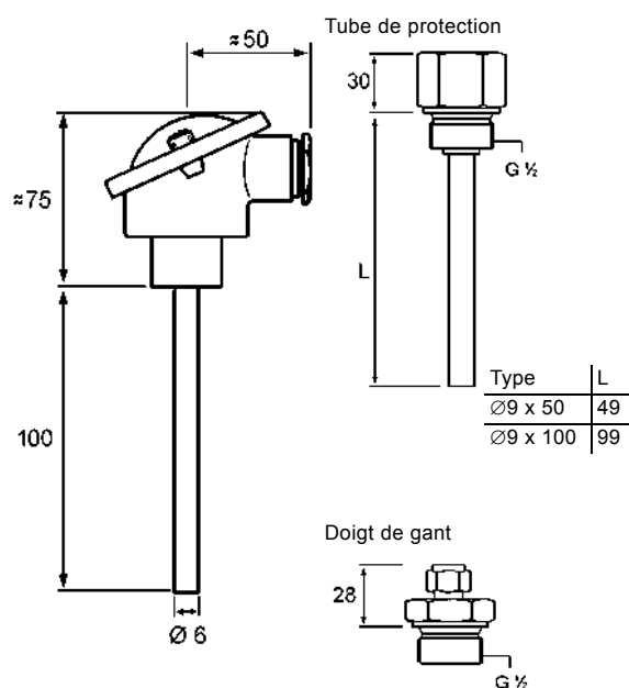
Fig. 114 Schémas cotés
