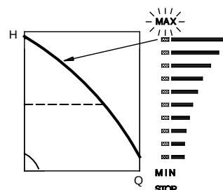
Fig. 44 Courbe maxi
