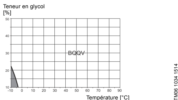
Fig. 8 Plage de service des garnitures mécaniques FKM
