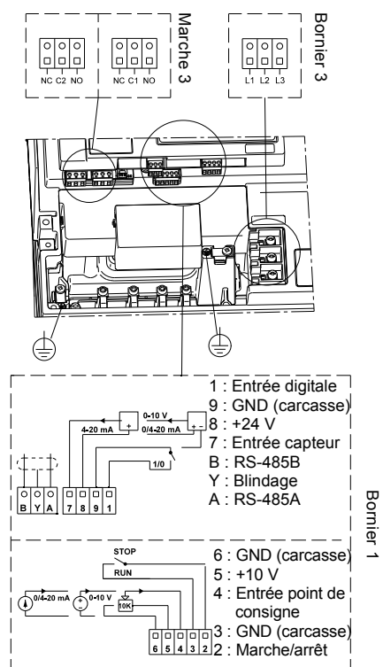
Fig. 109 Bornes de connexion
